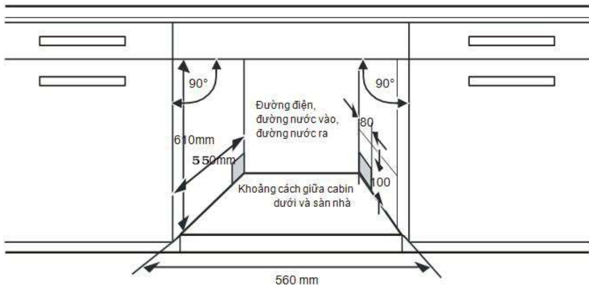
Hình minh họa kích thước tủ và vị trí lắp đặt máy rửa bát.
