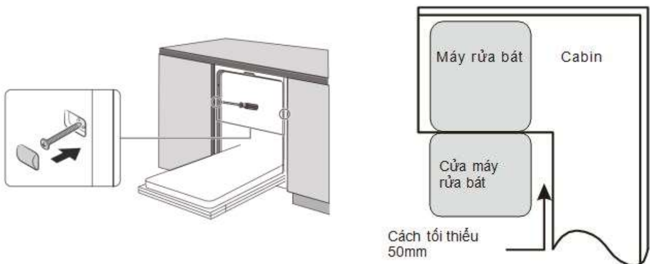
Lắp máy rửa bát vào tủ
